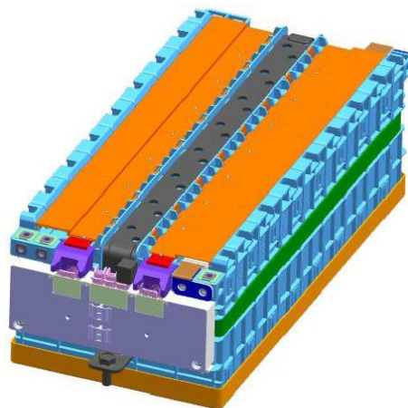
图 2 电池模组示意图
